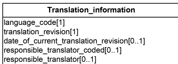
Figure 13 – Information de traduction (diagramme de classe UML)
