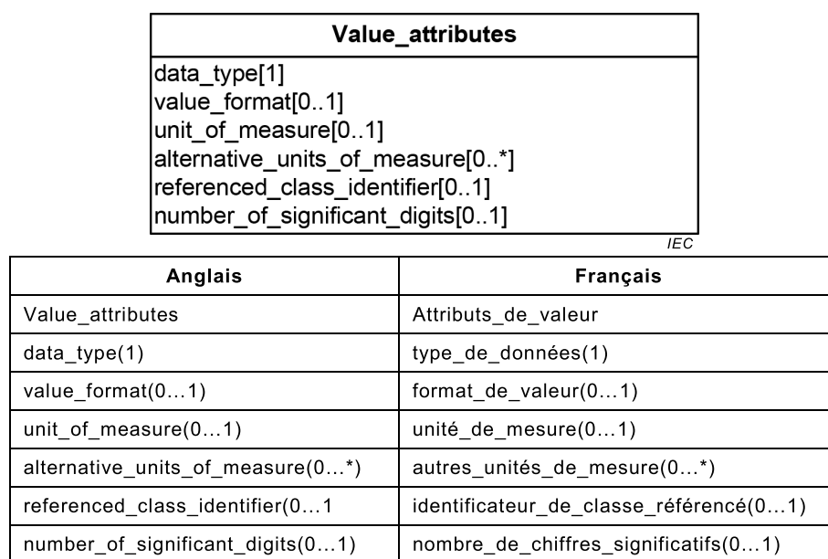
Figure 7 – Attributs de valeur (diagramme de classe UML)
